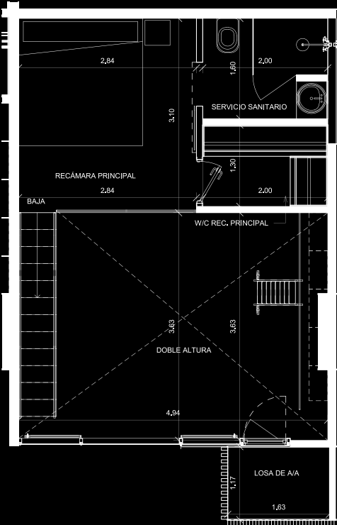
PLANTA ALTA
