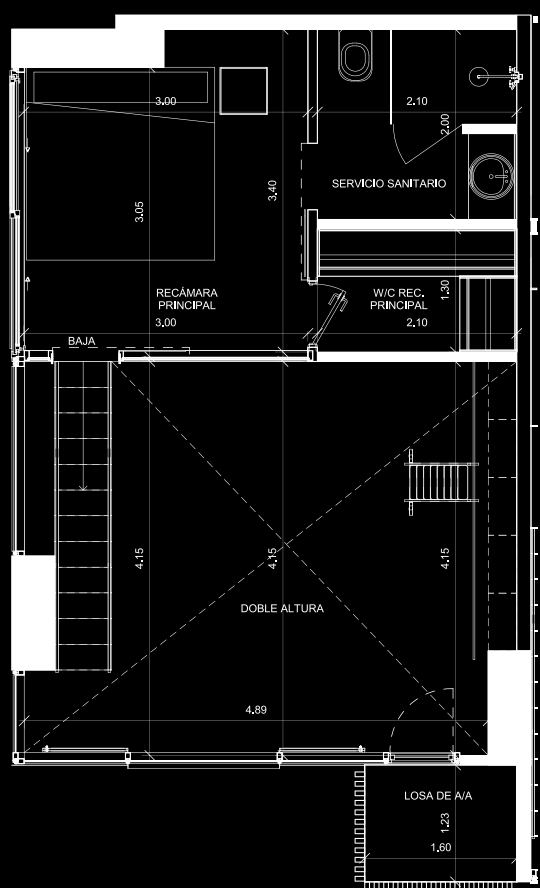
PLANTA ALTA
