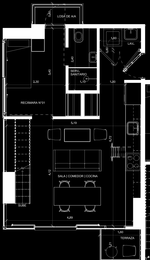
PLANTA BAJA
