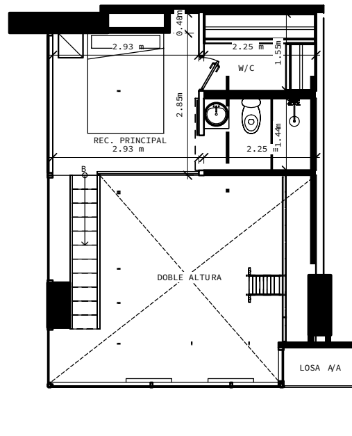
PLANTA ALTA
