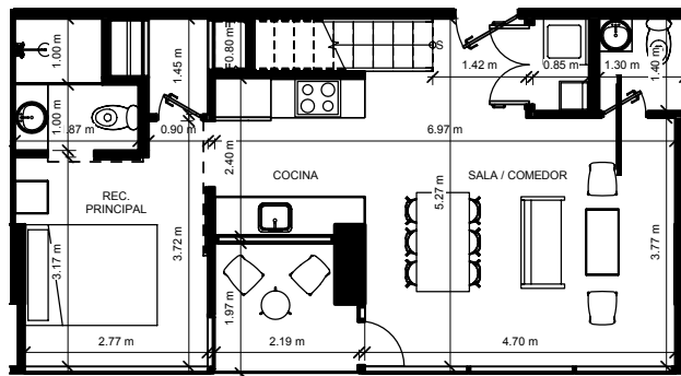
PLANTA BAJA
