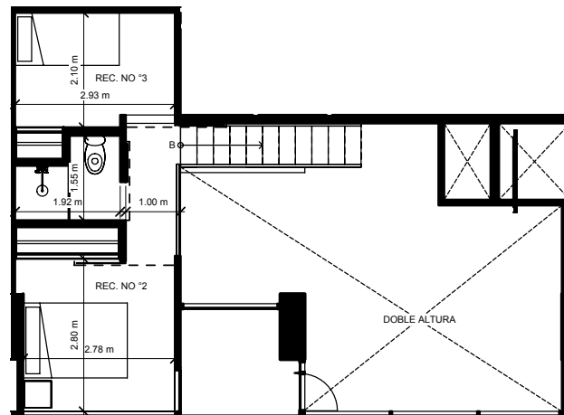
PLANTA ALTA
