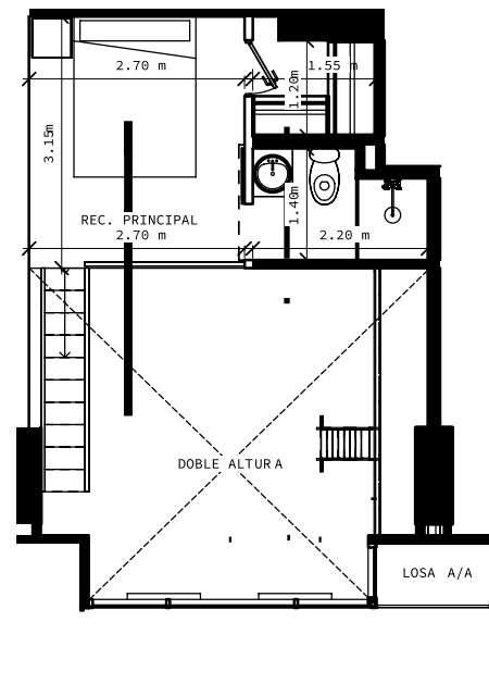
PLANTA ALTA
